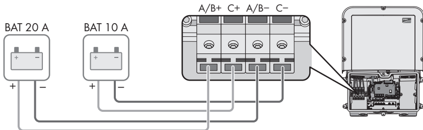
Figure 9 : Possibilités de raccordement (exemple)
