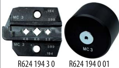
MC 3 Die Set
