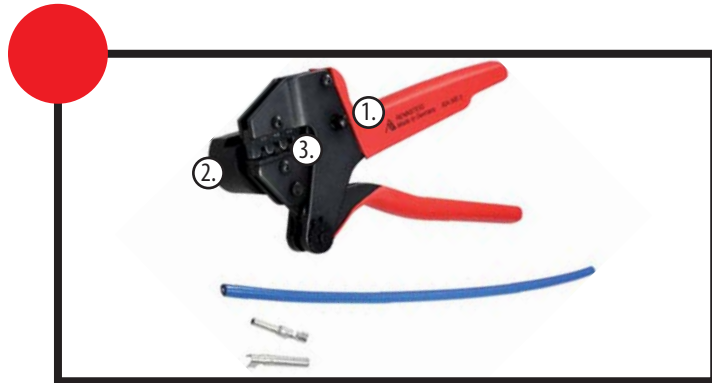
1. Tool 2. Locator 3. Die
