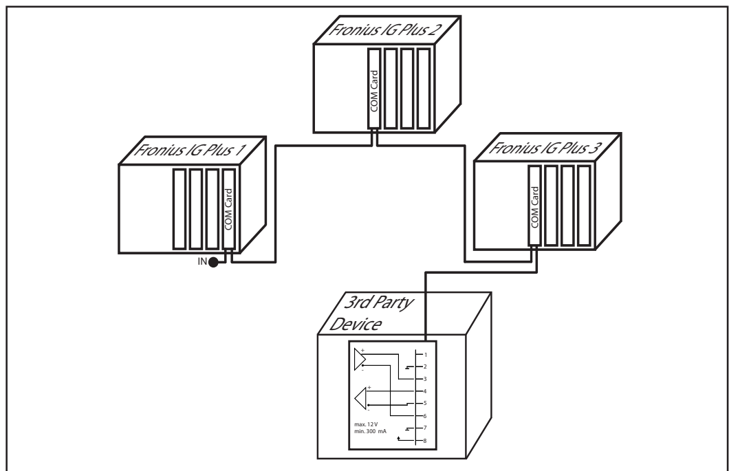
Possibile disposizione di sistema
