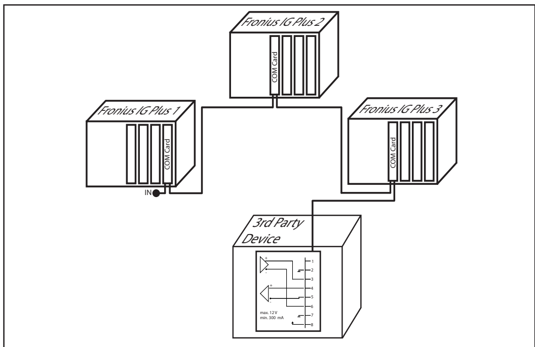
Mögliche Systemanordnung
